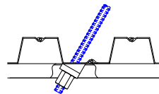
Schräger Einbau angular installation
