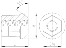
bombeli somun 55° dome nut 55°
