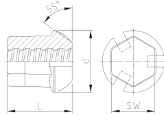
dolgu yuvalarına sahip bombeli somun 55° domed nut 55° with grout slots
