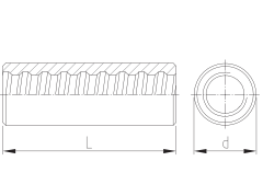
uzun kaplin coupler long
