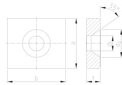
dikdörtgen ankraj plakası 55°, küçük anchor plate rectangular 55°, small
