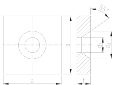
kare ankraj plakası 55° anchor plate square 55°
