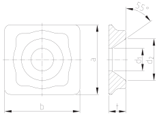
QR plakası QR plate
