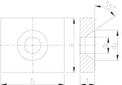
dikdörtgen ankraj plakası 55° anchor plate rectangular 55°
